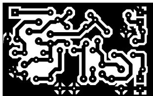
FOLIOKUVA JUOTOS- PUOLELTA KATSOTTUNA
