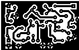
FOLIOKUVA KOMPONENTTI PUOLELTA KATSOTTUNA
