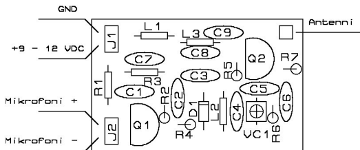
OSASIJOITTELUKUVA
